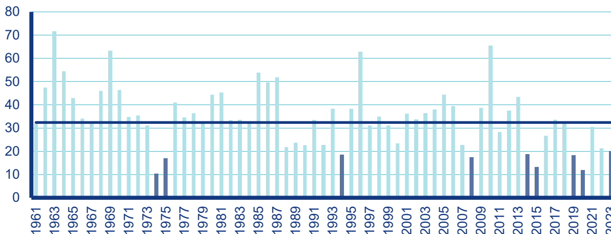
Obr. 2.23 Průměrný roční počet ledových dní na území ČR v období 1961–2023. Zvýrazněny jsou roky s počtem ledových dní 20 a nižším. Modrá příčka značí hodnotu dlouhodobého průměru za období 1991–2020.
