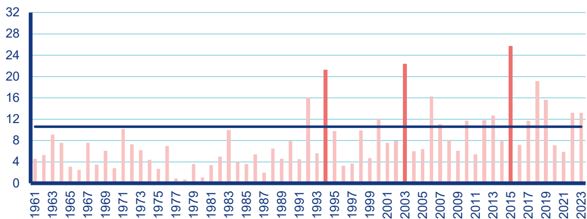
Obr. 2.22 Průměrný roční počet tropických dní na území ČR v období 1961–2023. Zvýrazněny jsou roky s počtem tropických dní 20 a vyšším. Modrá příčka značí hodnotu dlouhodobého průměru za období 1991–2020.
