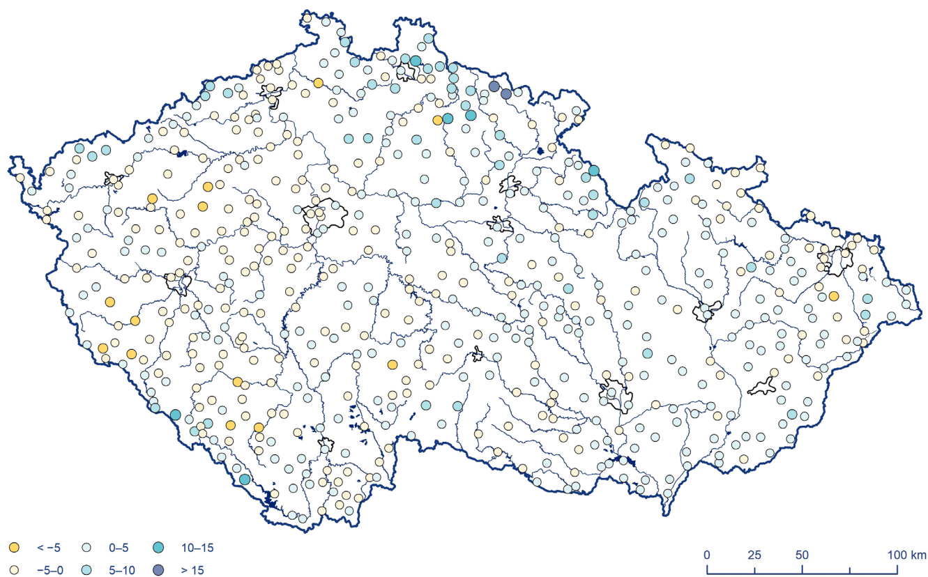
Obr. 3.11 Odchylka počtu dní s denním úhrnem srážek 10 mm a více v roce 2023 od dlouhodobého průměru 1991–2020.
