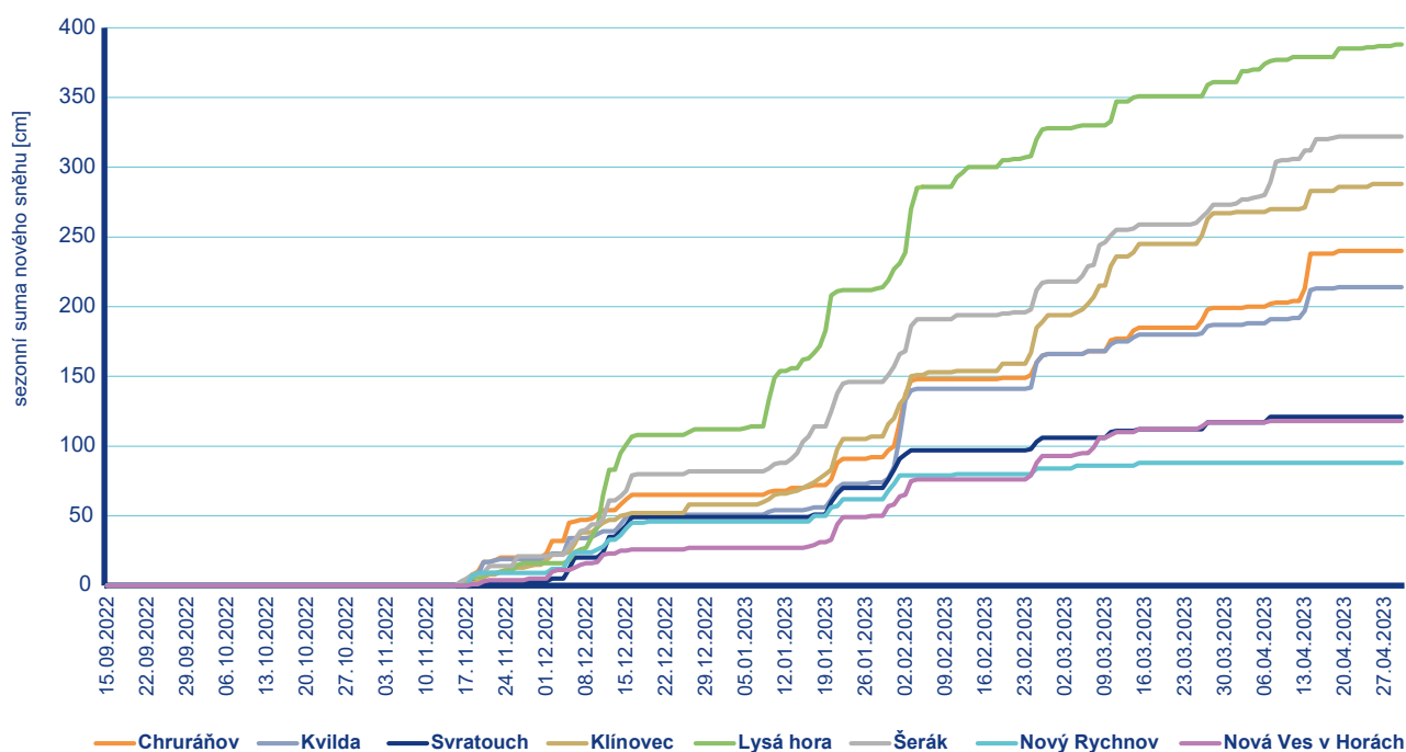
Obr. 4.4 Součtová křivka nového sněhu [cm] v sezoně 2022/2023 na vybraných stanicích.
