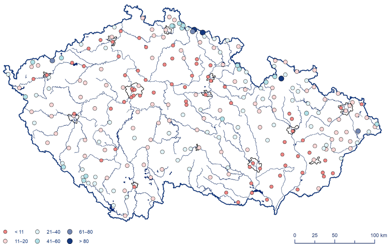
Obr. 2.15 Počet ledových dní (denní maximum teploty vzduchu < 0^{\circ}\text{C} ) v roce 2023.
