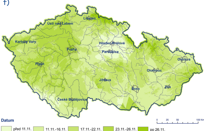
Obr. 8.2 Fenologické fáze břízy bělokoré v roce 2023 (vlevo) a odchylky jejich nástupů od průměru 1991–2020 (vpravo): a) rašení, b) první listy, c) plné olistění, d) počátek kvetení, e) konec kvetení, f) opad listů.
