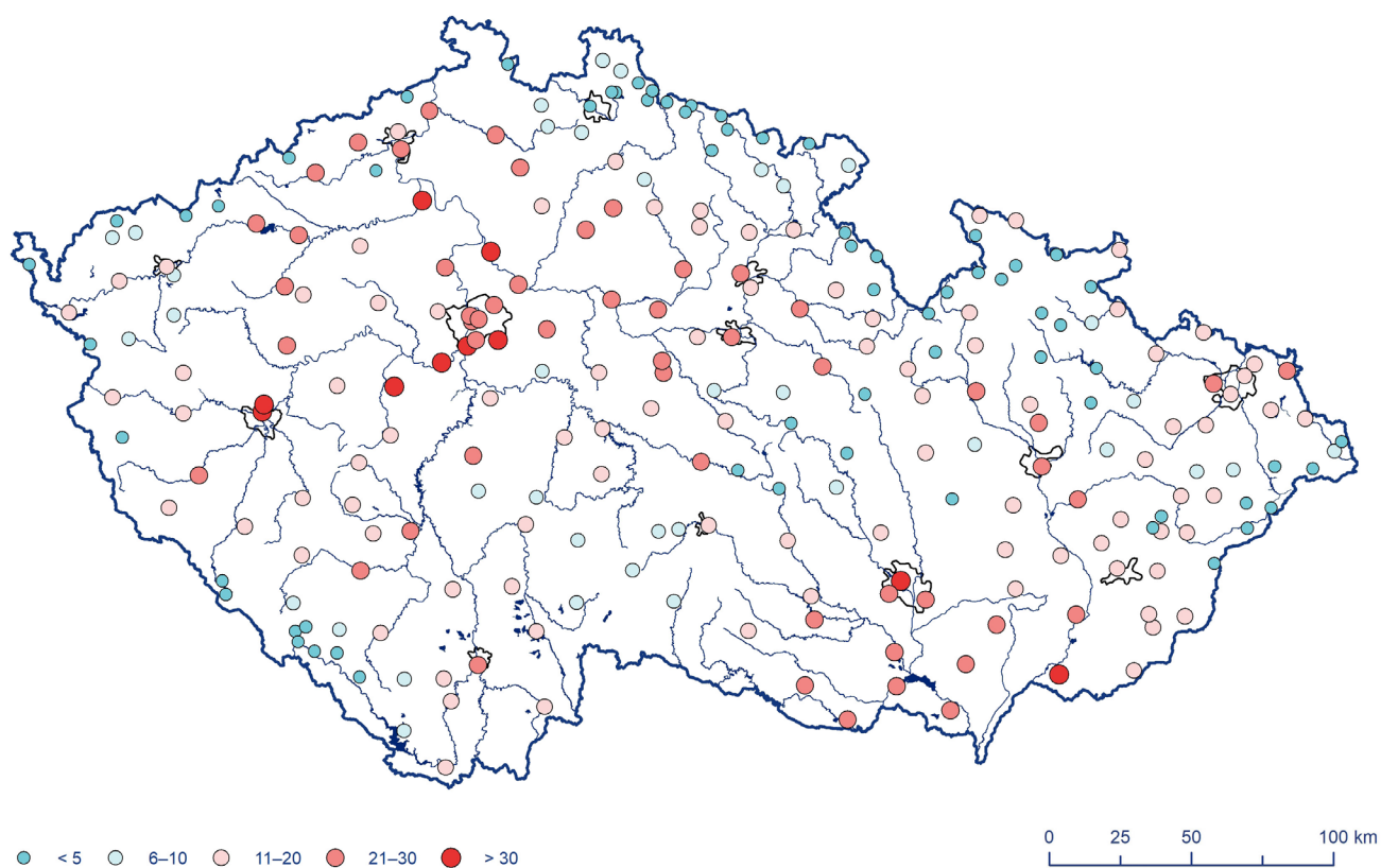
Obr. 2.19 Počet tropických dní (denní maximum teploty vzduchu \geq 30 °C) v roce 2023.
