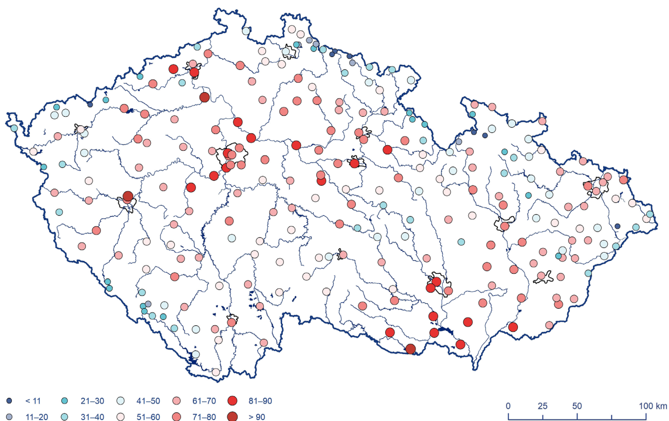
Obr. 2.17 Počet letních dní (denní maximum teploty vzduchu \geq 25\text{ °C} ) v roce 2023.
