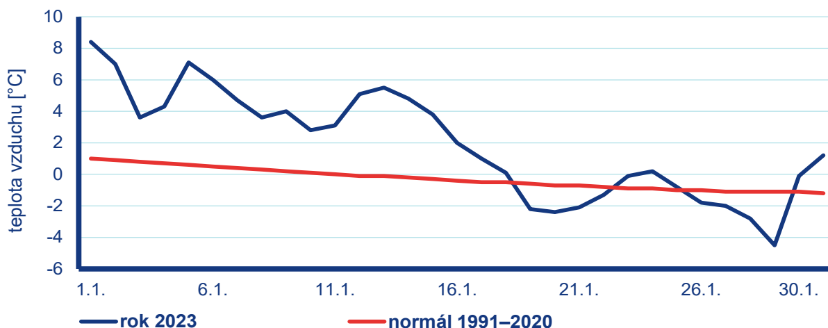
Obr. 7.1 Průběh průměrné denní teploty vzduchu na území ČR v lednu 2023 ve srovnání s normálem 1991–2020.
