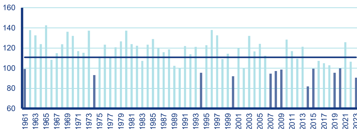
Obr. 2.24 Průměrný roční počet mrazových dní na území ČR v období 1961–2023. Zvýrazněny jsou roky s počtem mrazových dní 100 a nižším. Modrá příčka značí hodnotu dlouhodobého průměru za období 1991–2020.
