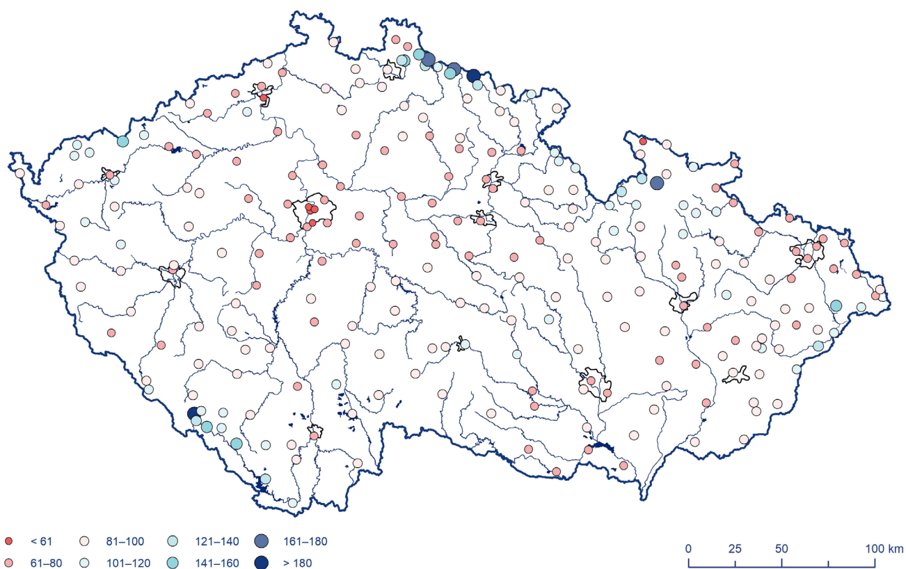
Obr. 2.13 Počet mrazových dní (denní minimum teploty vzduchu < 0^{\circ}\text{C} ) v roce 2023.
