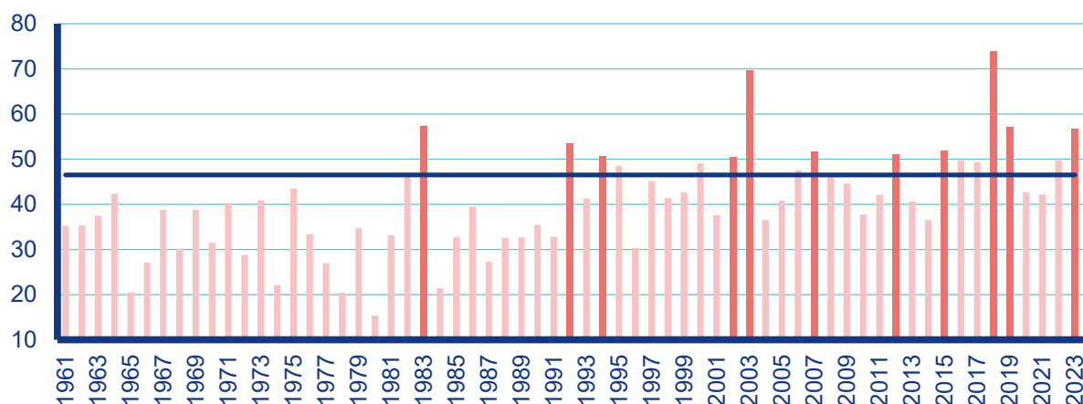
Obr. 2.21 Průměrný roční počet letních dní na území ČR v období 1961–2023. Zvýrazněny jsou roky s počtem letních dní 50 a vyšším. Modrá příčka značí hodnotu dlouhodobého průměru za období 1991–2020.
