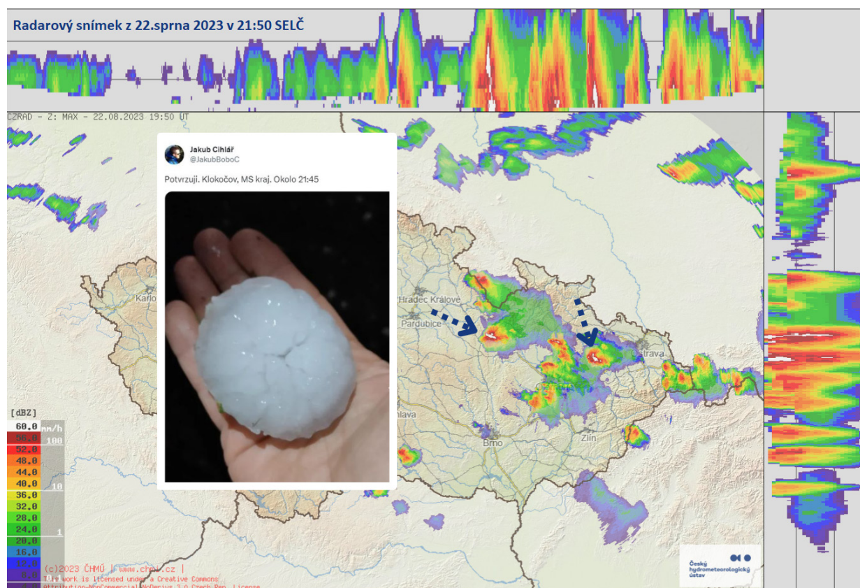
Obr. 7.6 Radarový snímek z 22. srpna 2023 v 21:50 SELČ.
