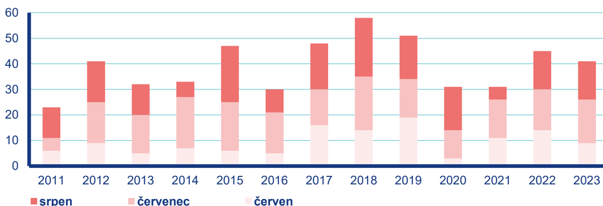
Obr. 2.6 Počet tropických dní zaznamenaných v letní sezoně let 2011–2023. Tropický den je uvažován, pokud nastal alespoň na jedné stanici standardní sítě ČHMÚ.
