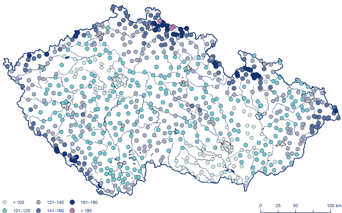
Obr. 3.8 Počet dní s denním úhrnem srážek 1 mm a více v roce 2023.
