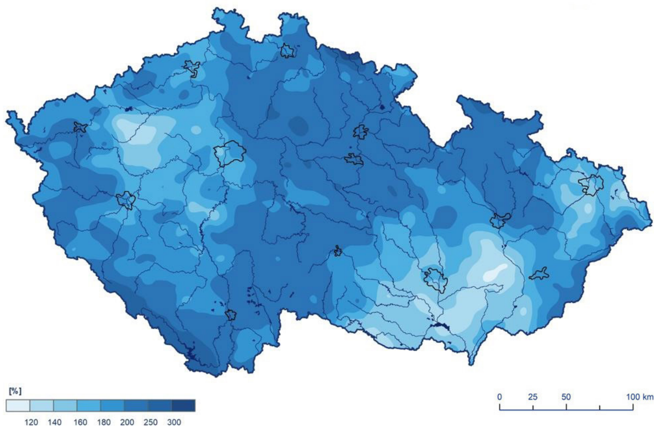
Obr. 7.11 Měsíční úhrn srážek na území ČR v listopadu 2023 v % normálu.
