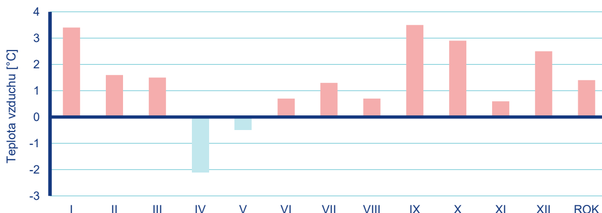
Obr. 2.5 Odchylka průměrné měsíční teploty vzduchu [°C] na území ČR od normálu 1991–2020 v jednotlivých měsících roku 2023.
