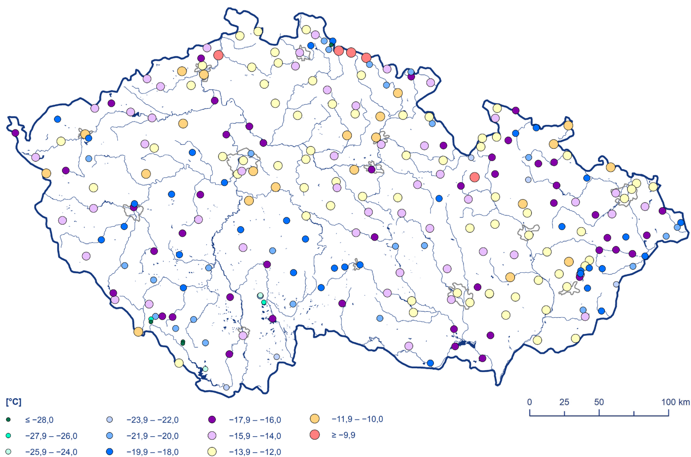
Obr. 2.25 Nejnižší minimální přízemní teplota vzduchu [°C] v ČR v roce 2023.
