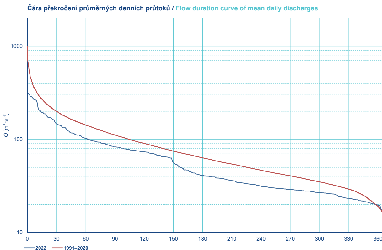
Obr. I.2.2 Průměrné denní průtoky (tabulka, hydrogram a čára překročení) za rok 2022 pro vodoměrnou stanici Kostelec nad Labem na Labi.
