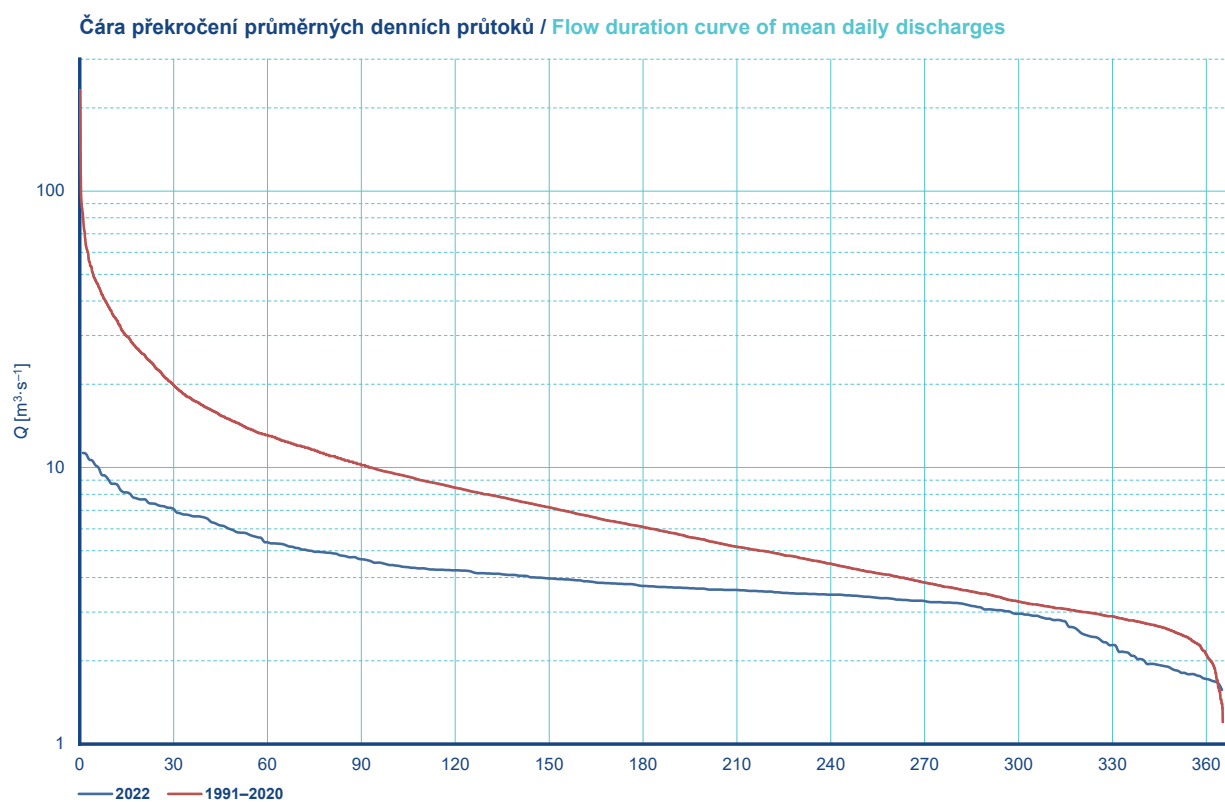
Obr. I.2.11 Průměrné denní průtoky (tabulka, hydrogram a čára překročení) za rok 2022 pro vodoměrnou stanici Ivančice na Jihlavě.
