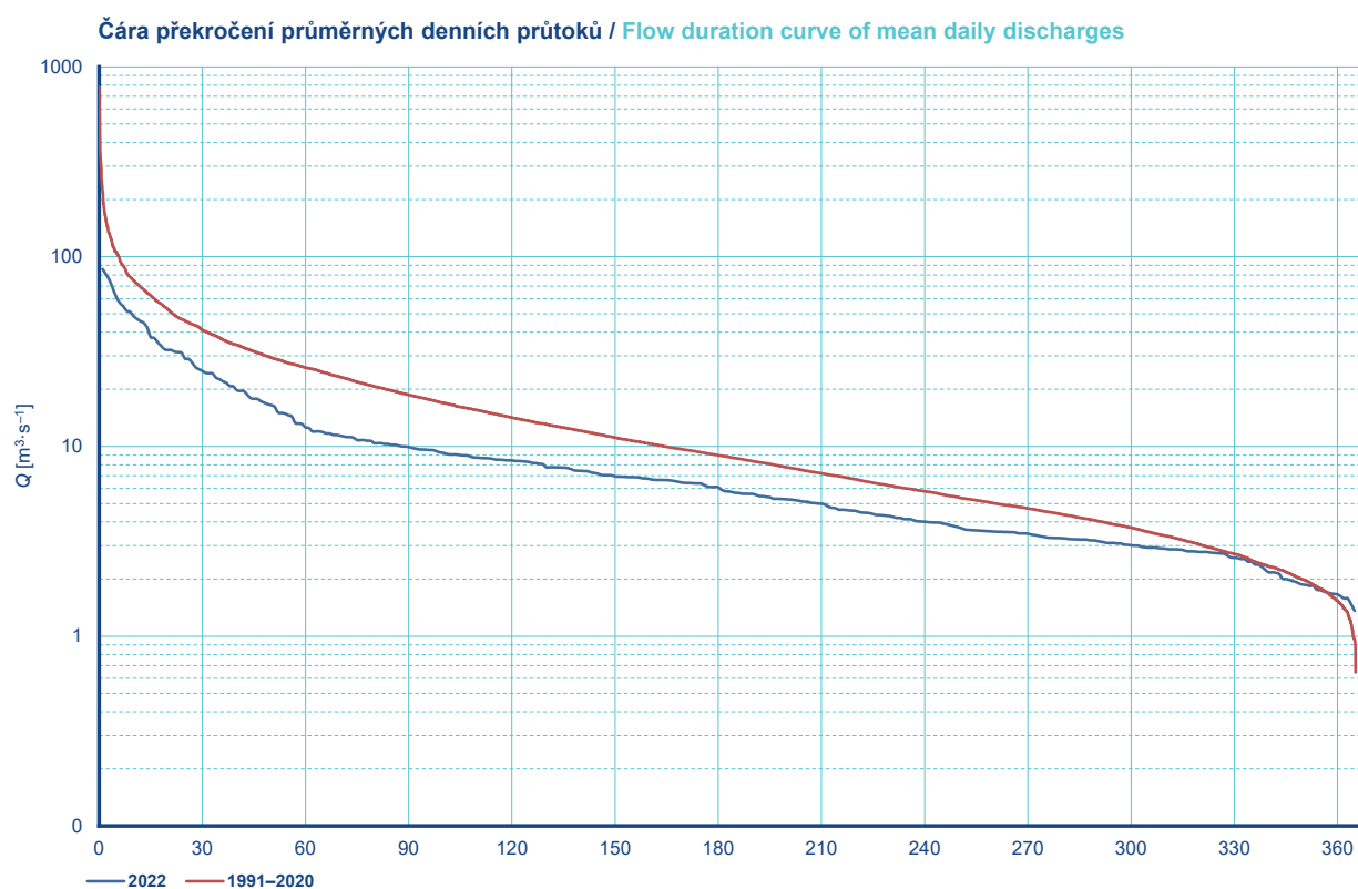
Obr. I.2.9 Průměrné denní průtoky (tabulka, hydrogram a čára překročení) za rok 2022 pro vodoměrnou stanici Dluhonice na Bečvě.
