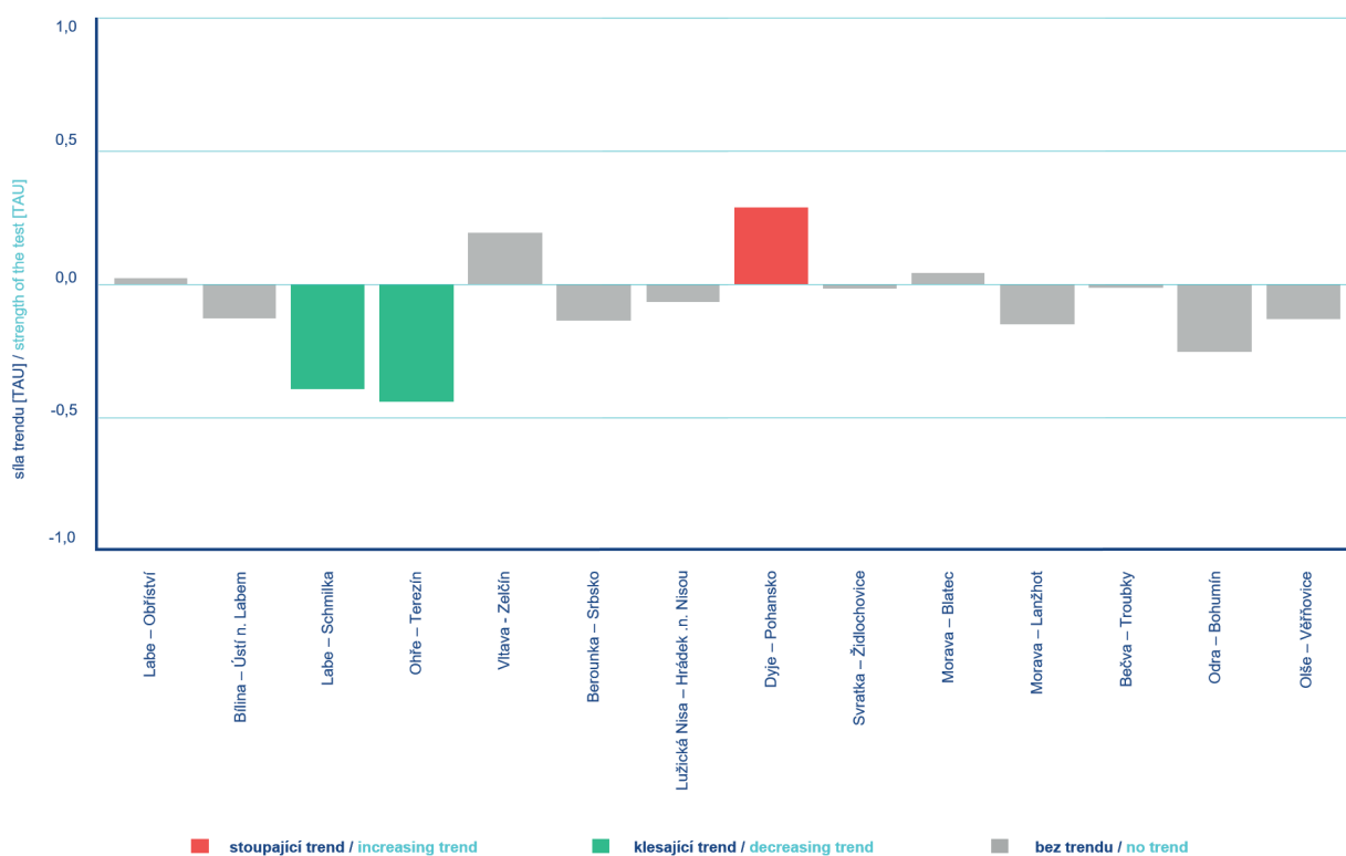
Obr. III.3.16 Přehled profilů s rostoucím a klesajícím trendem koncentrací benzo[ghi]perylenu v sedimentovatelných plaveninách.
