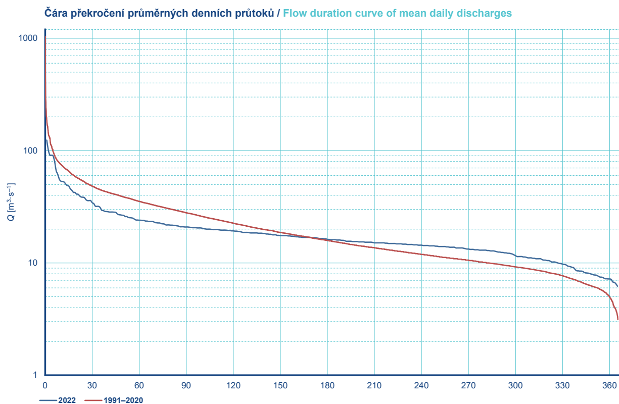
Obr. I.2.3 Průměrné denní průtoky (tabulka, hydrogram a čára překročení) za rok 2022 pro vodoměrnou stanici Písek na Otavě.
