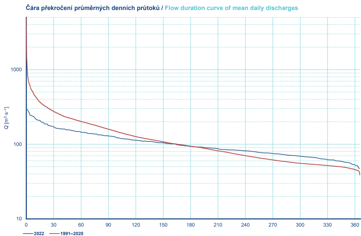
Obr. I.2.5 Průměrné denní průtoky (tabulka, hydrogram a čára překročení) za rok 2022 pro vodoměrnou stanici Praha-Chuchle na Vltavě.
